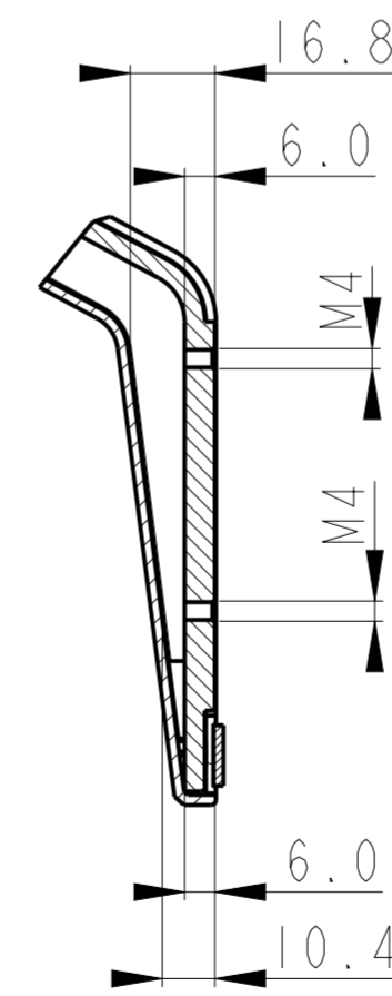
SECTION V-V
